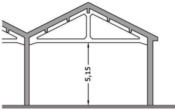
SEZIONE A-A
